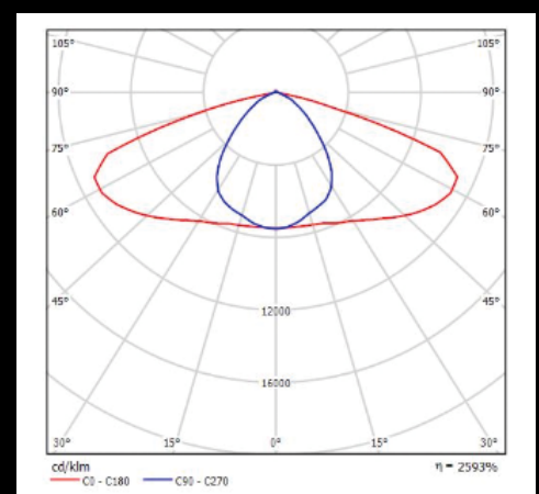
Abstrahlcharakteristik.
